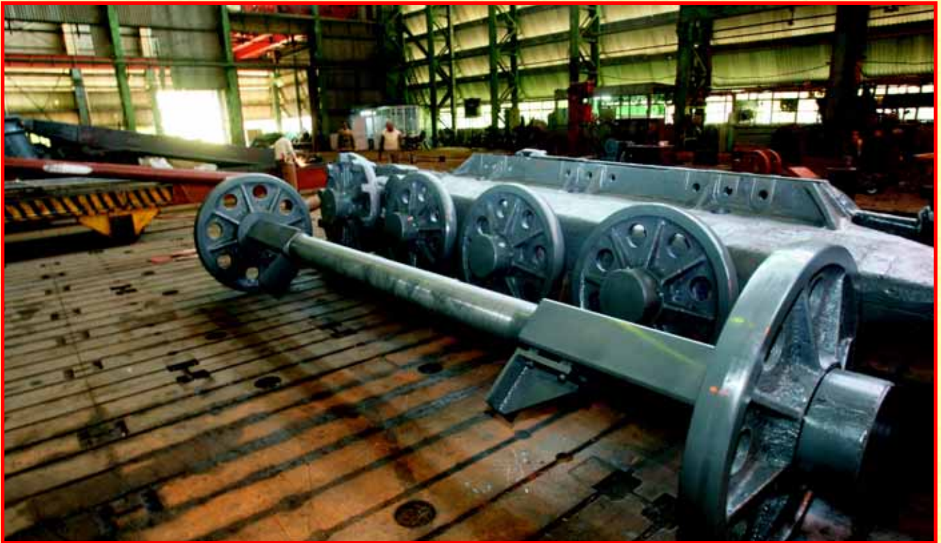
5 क्युबिक मीटर शावेल के स्पेयर्स
